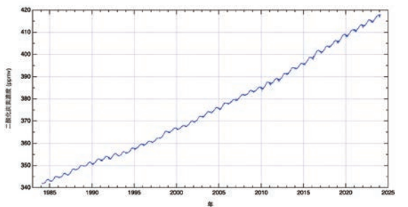
昭和基地で観測された大気中二酸化炭素濃度の変動
