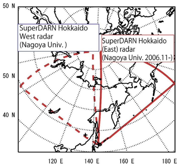
左図: SuperDARN 北海道-陸別第一レーダー(実線)および第二レーダー(点線)の視野図。
